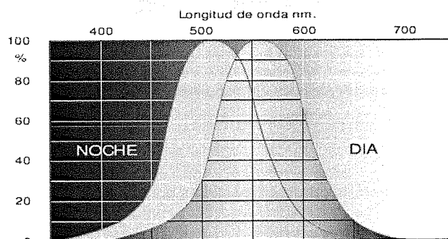
Figura 4. Curva de sensibilidad del ojo a las radiaciones monocromáticas.
